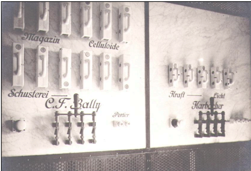
Schalttafel bei der EGS, 1896
